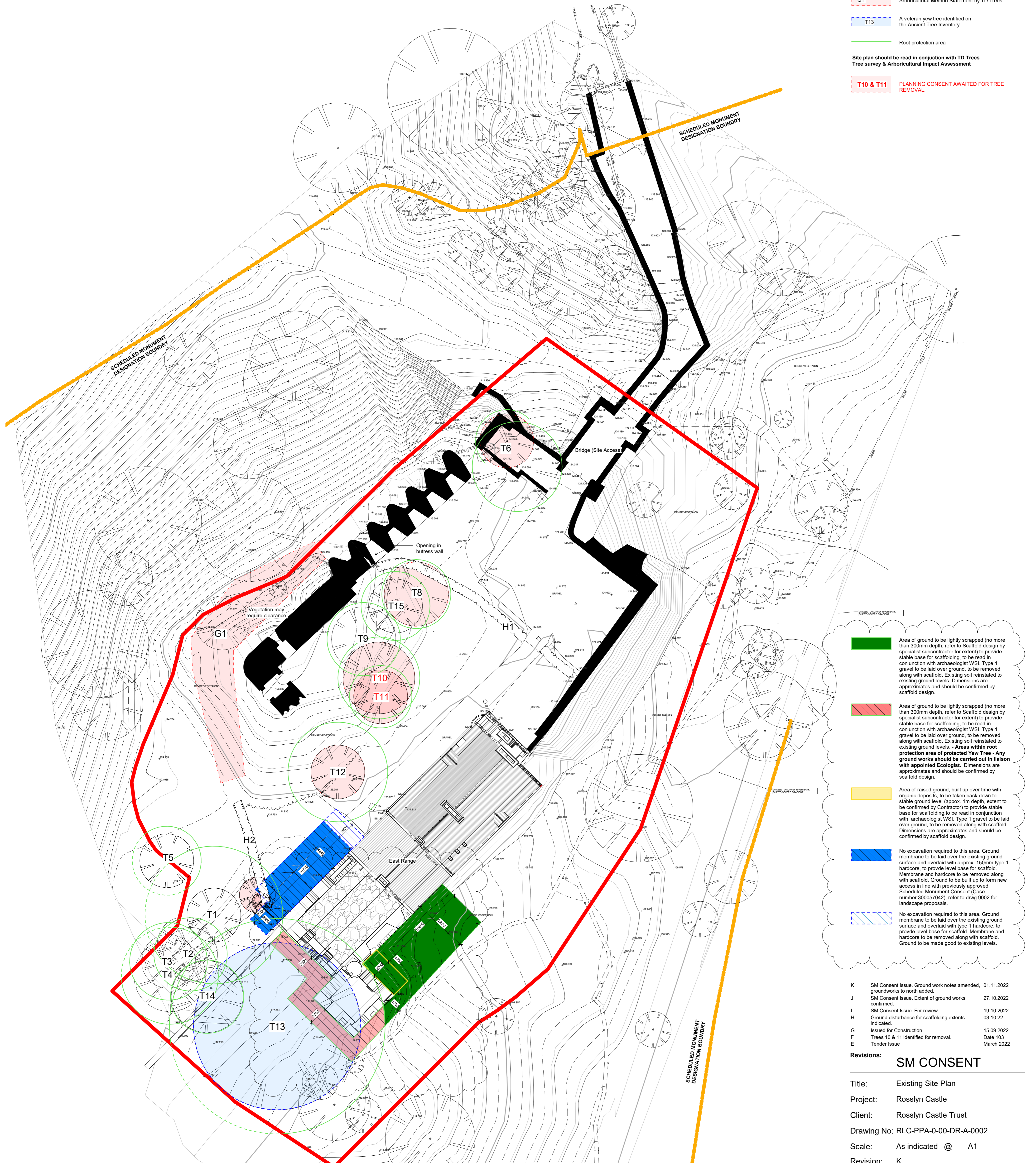
1 Site Plan - Existing 1 : 200
