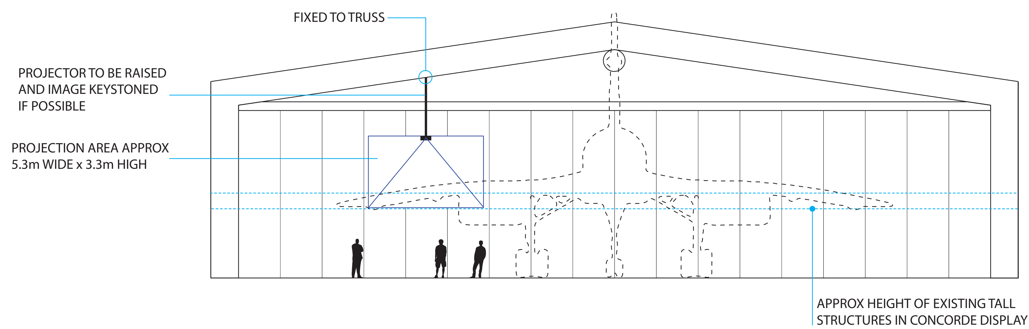
ELEVATION A-A
